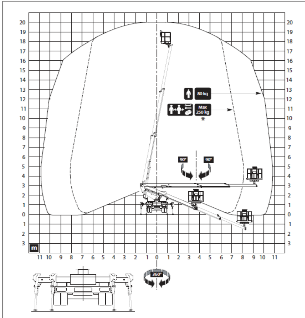
Schema werkomgeving met uitgeschoven stabilisatiearmen
