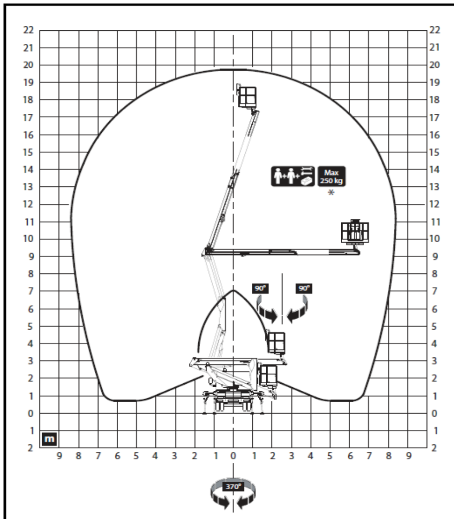
Schema werkomgeving met uitgeschoven stabilisatiearmen
