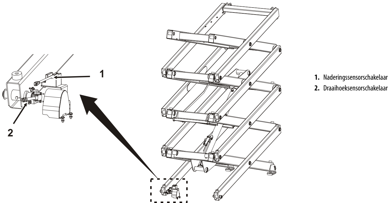
Figuur 2-4. Plaats van afslagschakelaars
