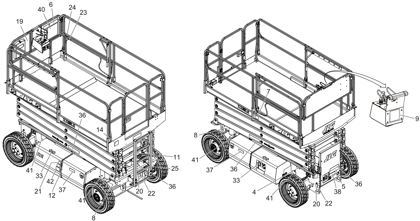
Figuur 3-6. Plaats van stickers (CE/AUS)
