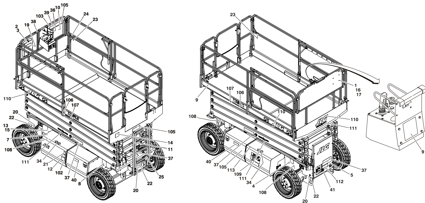
Figuur 3-4. Plaats van stickers (ANSI)
