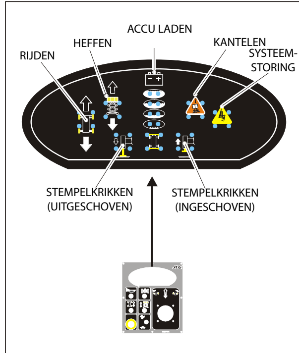
Figuur 3-3. Indicatorpaneel
