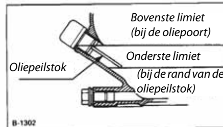
Kubota-motor OC60-D – locatie oliepeilstok en aftapstop
