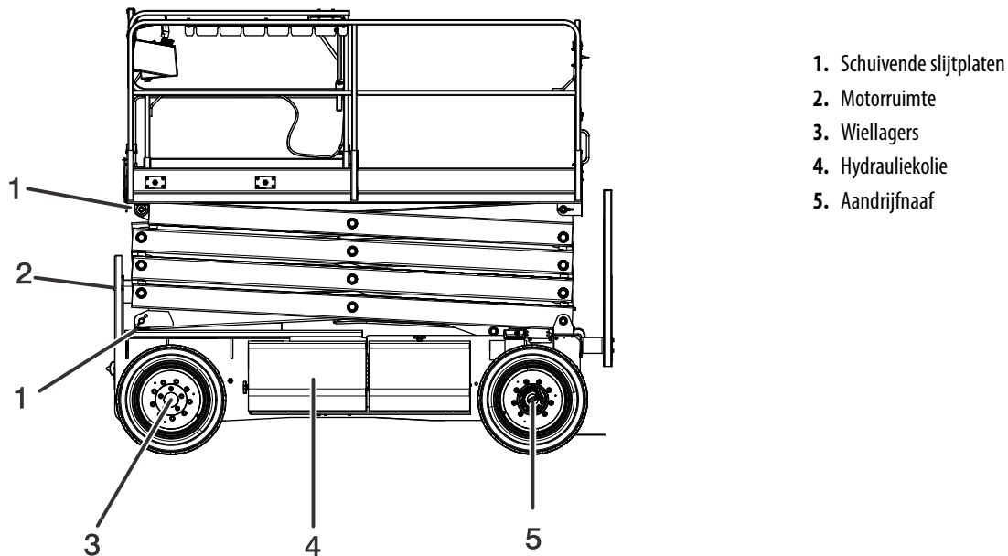
Figuur 6-3. Schema voor onderhoud en smering door machinist
