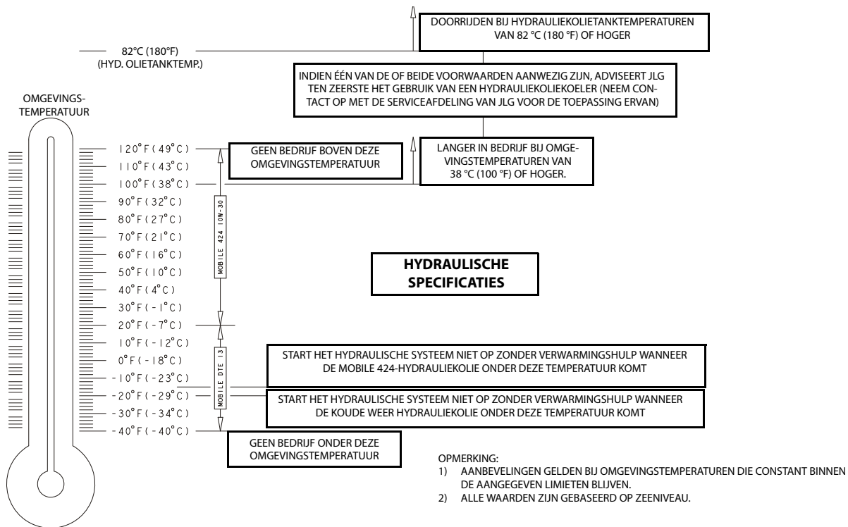
Figuur 6-2. Specificaties motorbedrijfstemperatuur – (Kubota) Blad 2 van 2
