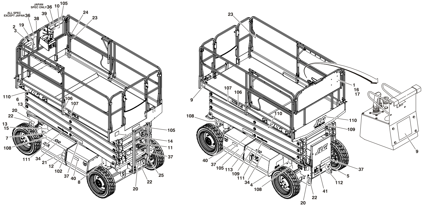
Figuur 3-5. Plaats van stickers (export ANSI)
