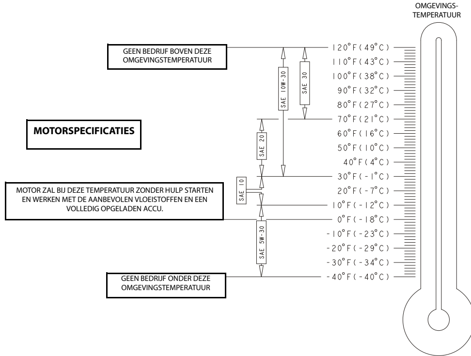
Figuur 6-1. Specificaties motorbedrijfstemperatuur – (Kubota) Blad 1 van 2
