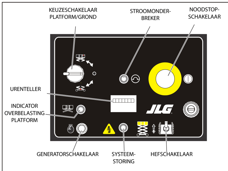
Figuur 3-1. Grondbedieningsstation
