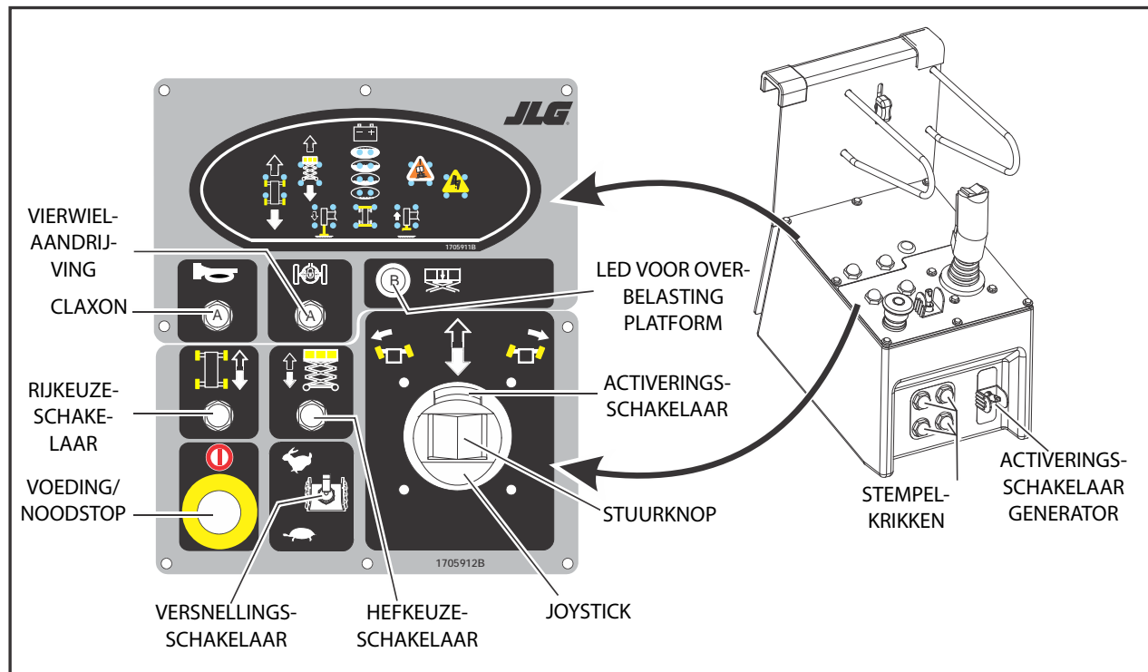
Figuur 3-2. Platformbedieningsstation
